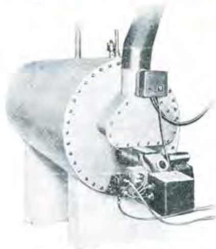
Equipo auto-bloque del generador para el servicio de agua caliente
